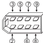
Колодка МК вид спереди, со стороны контактов
